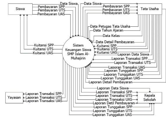
Gambar 2. DFD Konteks
